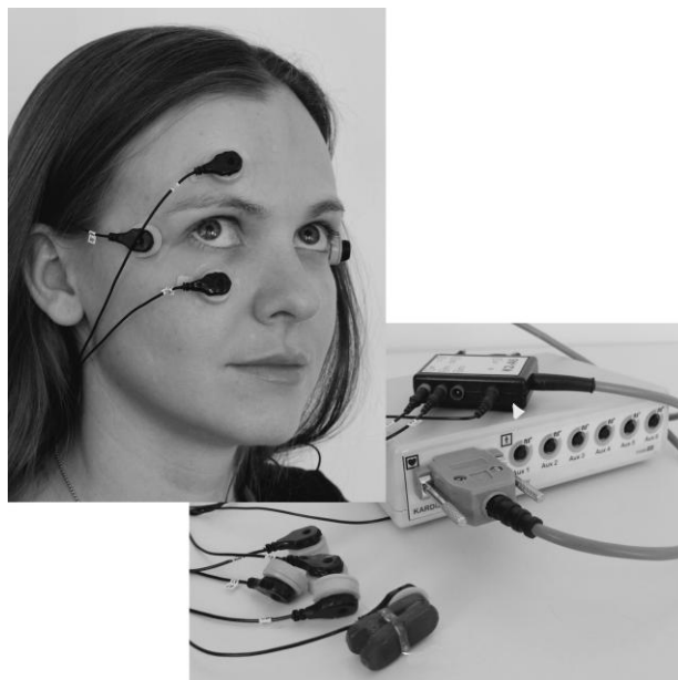
Рис. 3. Установка электродов при регистрации электроокулограммы; полиграфический усилитель kardi-2 с набором электродов (Центр экспериментальной психологии МГППУ)
